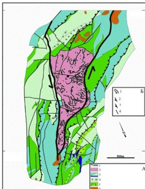
Рисунок 1 – Геологическая схема месторождения Сукари (А: 1 – Кварцевые жилы; 2 – Гранит- порфир; 3 – Андезиты и их туфы; 4 – Конгломераты; 5 – Андезито-базальты и их подушечные лавы; 6 – Габбро; Б: 1 – Сдвиги; 2 – Надвиги; 3 – Сбросы; 4 – Трещины)
