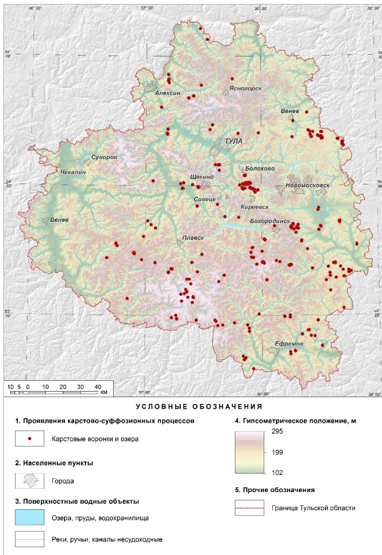
Рисунок 1 – Карта проявлений карстово-суффозионных процессов на территории Тульской области
