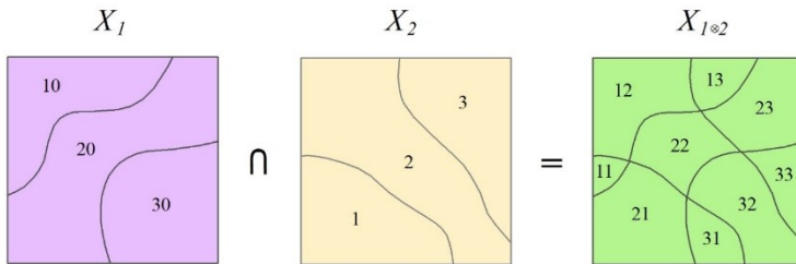
Рисунок 2 – Схема получения сложных факторов, определяющих пространственное распределение проявлений карстово-суффозионных процессов
